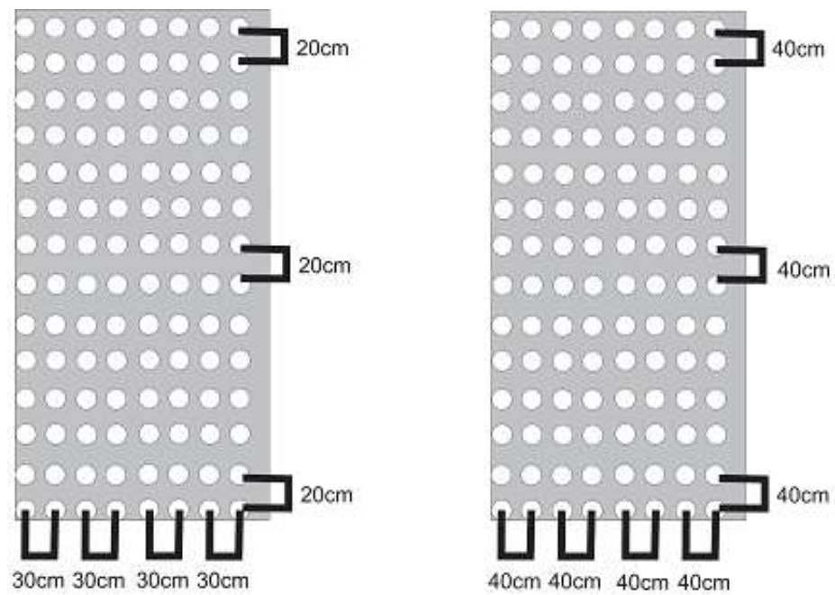
Gambar 7. Uji Jarak dengan Sistem Knock Down
