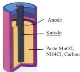
Gambar 3. Baterai
